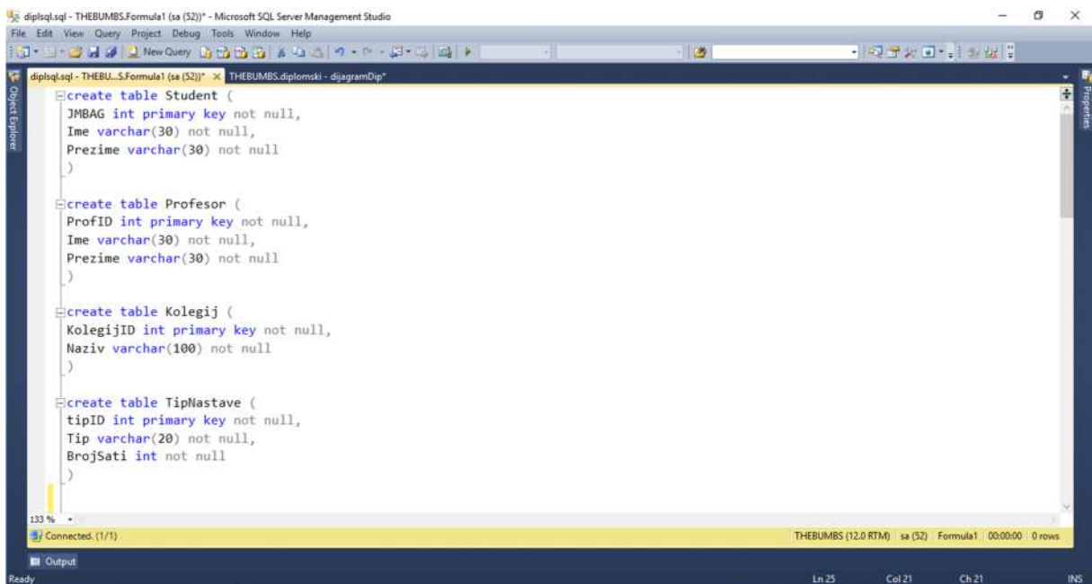
Slika 9. Kreiranje tablica
