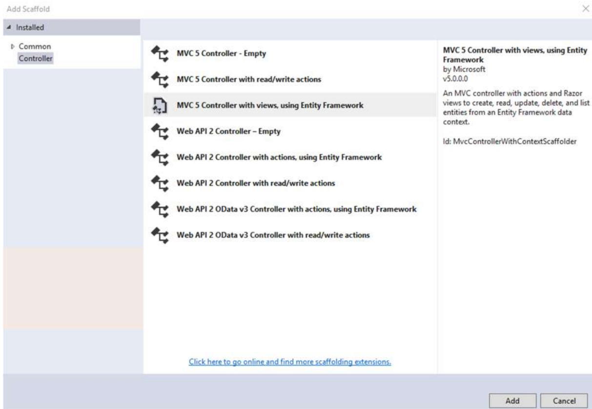
Slika 33. Odabir scaffold-a
