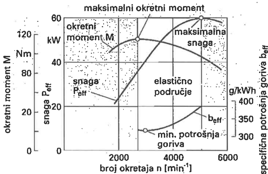
Slika 1. Karakteristike 4T Otto-motora
