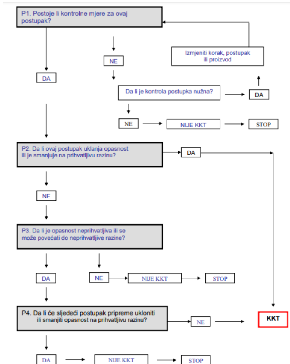
Slika 9: Stablo odlučivanja
