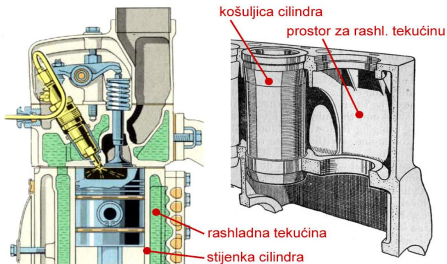
Slika 3. Cilindar bez košuljice lijevo i s košuljicom desno
