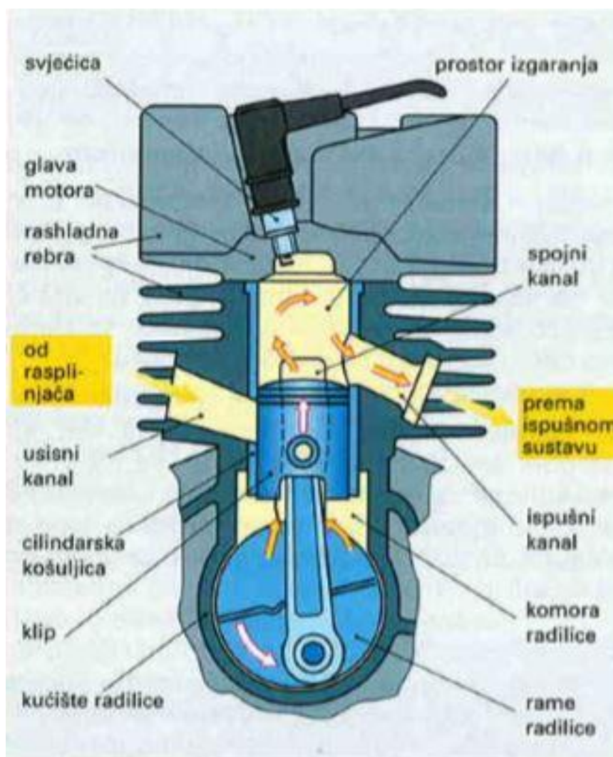
Slika 12: Dvotaktni Otto motor
