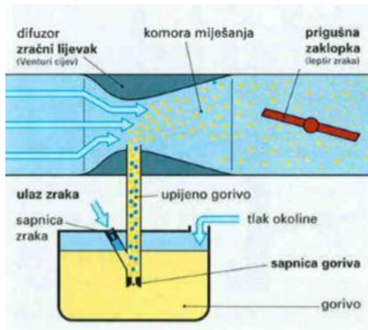
Slika 16: Rasplinjač
