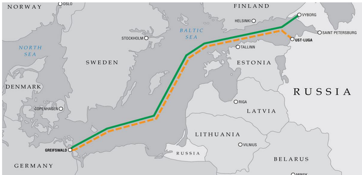
Slika 9. Postojeći plinovod Sjeverni tok 1 i planirani Sjeverni tok 2.
