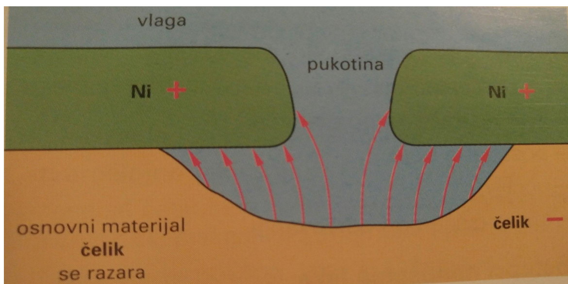
Slika 11, nepravna zaštita
