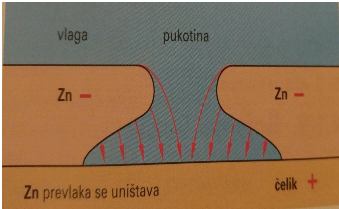
Slika 10, prava zaštita
