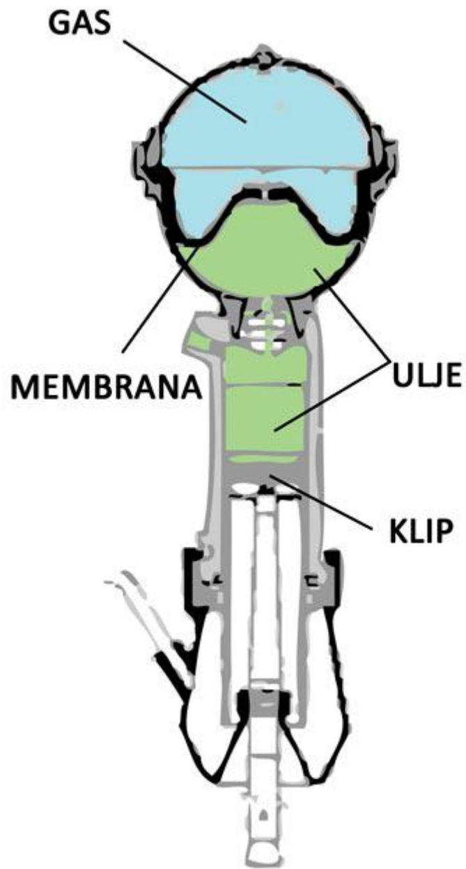
Slika 20, hidropneumatska opruga
