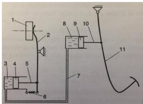
Slika 14. Hidraulični uređaj za isključivanje spojke
