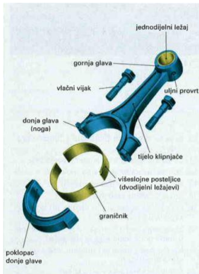
Slika 4: Dvodijelna klipnjača
