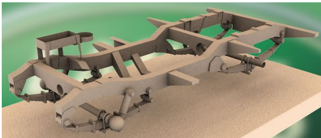
Slika 1. Odvojena karoserija
