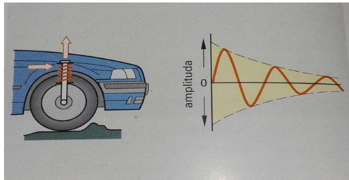
Slika 3. Slobodne, vibracije s prigušenjem
