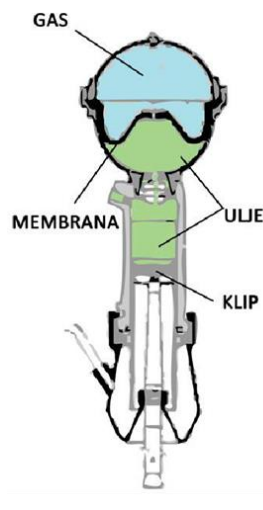
Slika 8. Hidropneumatska opruga
