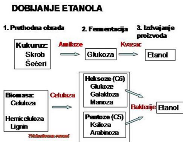
Slika 4. Dobivanje etanola.
