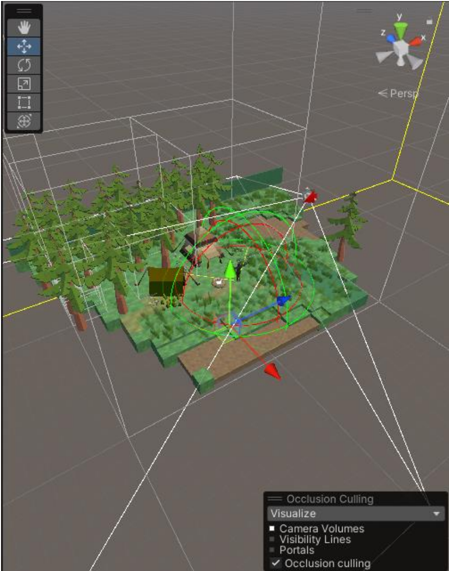
Slika 27- Primjer Occlusion-a
