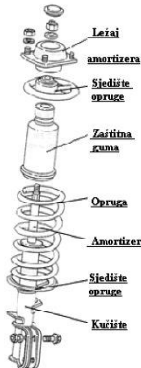
Slika 20.. Amortizer
